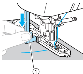
① Levier de boutonsnières
